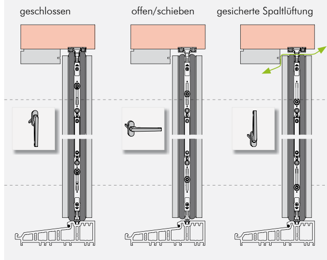
Bedienung und Funktionalität – bekannte Griffstellungen und Spaltlüftung
