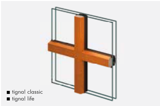
Einseitig aufgesetzte Trapezfalzsprosse/Alu-Sprosse im Scheibenzwischenraum (28 mm)
